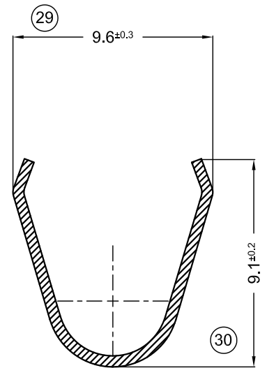
SECC. A-A
